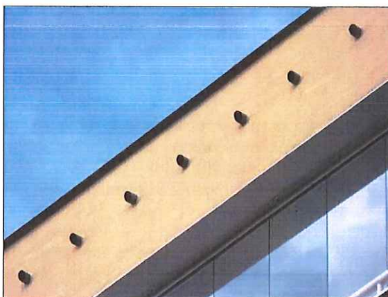
Ukázka nesprávného provedení opatření, trubky vyčnívají spodními okraji ze zateplené fasády a jsou pro roryse jen obtížně překonatelnou překážkou
